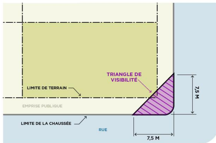
Figure 15. Triangle de visibilité d'un terrain résidentiel
